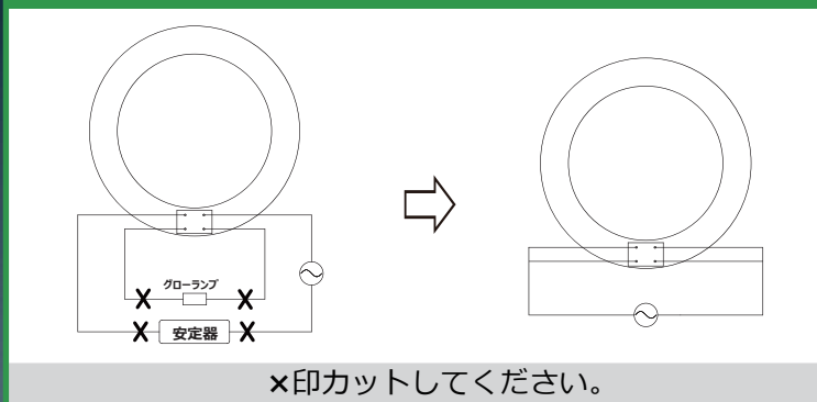
結線図 コンパクト蛍光灯 FCL代替 (電源直結タイプ)
