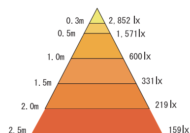
ACSQ(5700K)_1106mm 直下照度
