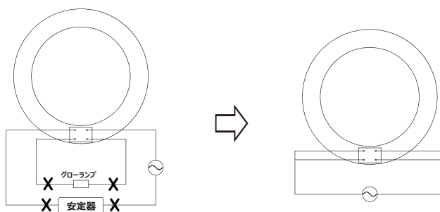
結線図 コンパクト蛍光灯 FCL代替 (電源直結タイプ)
